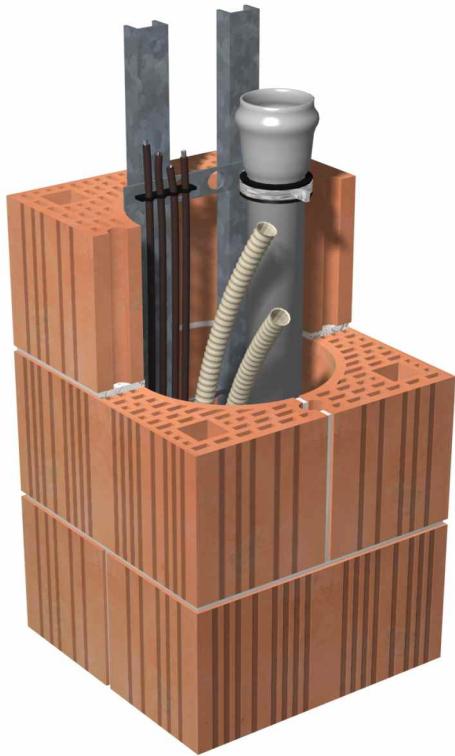
Ventilační průduch (cihla)
